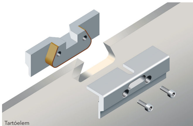
Tartóelem
