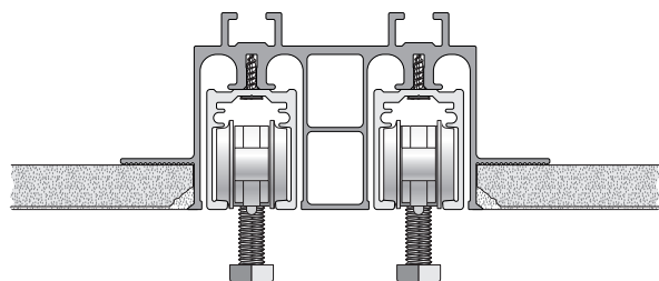
KÉTPÁLYÁS - MENNYEZETI SÍN
