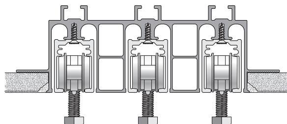
HÁROMPÁLYÁS - MENNYEZETI SÍN
