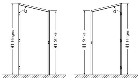
FELSŐ KERESZTTARTÓVAL
