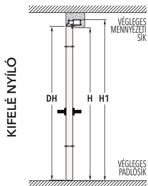
FELSŐ KERESZTTARTÓVAL
