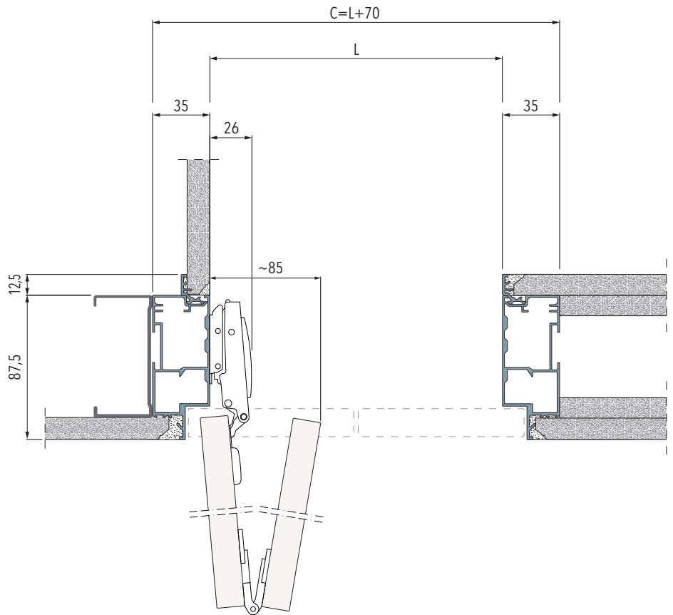
BIFOLD KIVITEL
